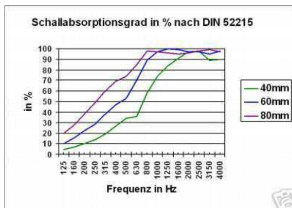
Bild: Schallabsorptionsgrad von Melaminharzschaumplatten verschiedener Dicken
